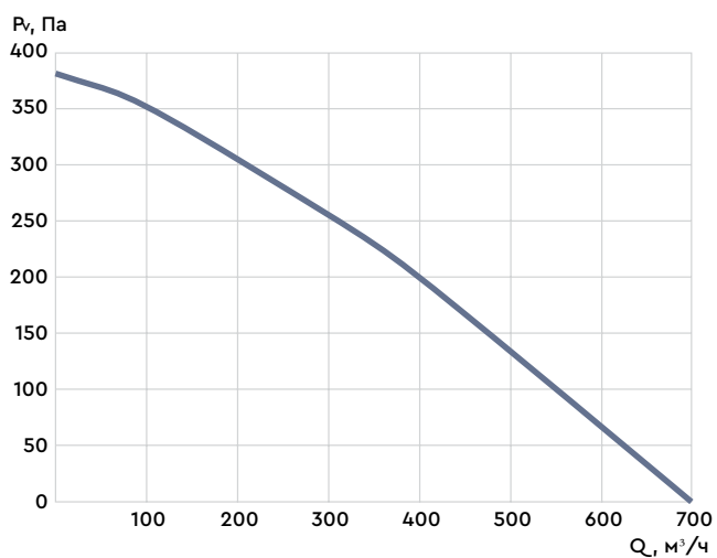
VRK PatAIR-K-160
