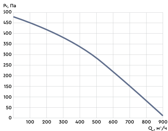
VRK PatAIR-K-200
